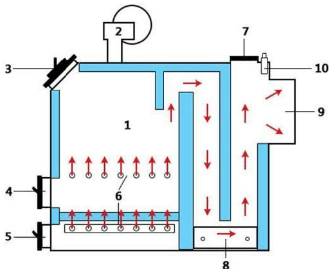
рис. 1 Конструкция котла
